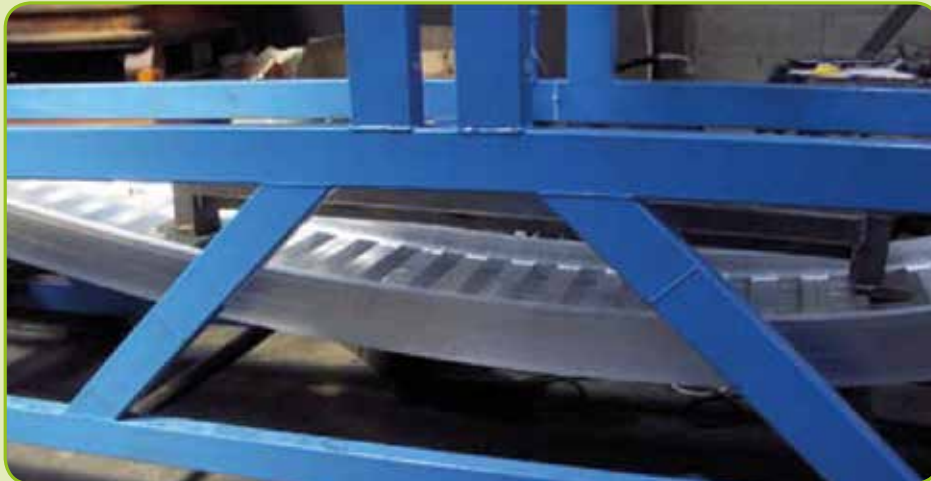
Rampa sottoposta a rottura.
